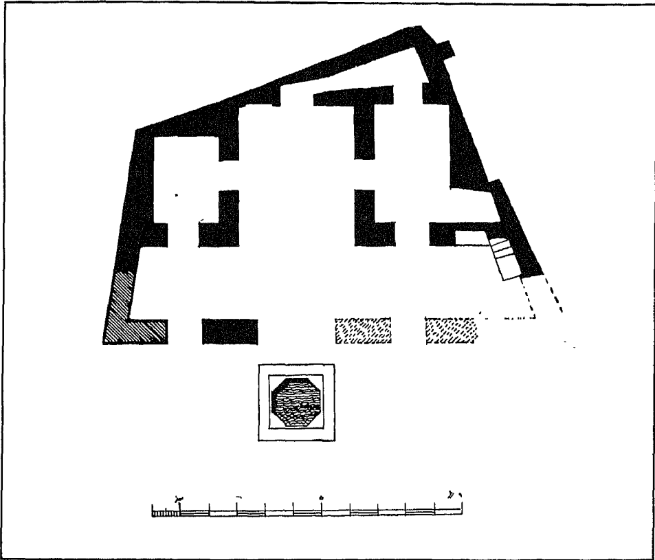
شكل (٥) البيت الطولونى الأول، مسقط أفقى، عن فريد شافعى.
